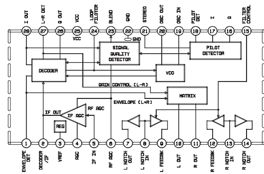
IC22 : MC13022DW
