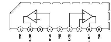
IC32 : MC4558S
