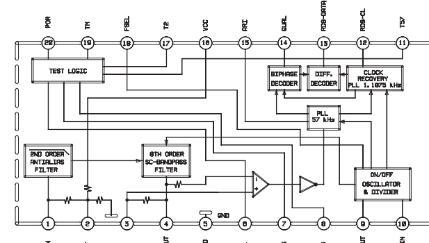
IC80 : TDA7330BD
