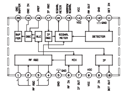
IC21 : LA1135
