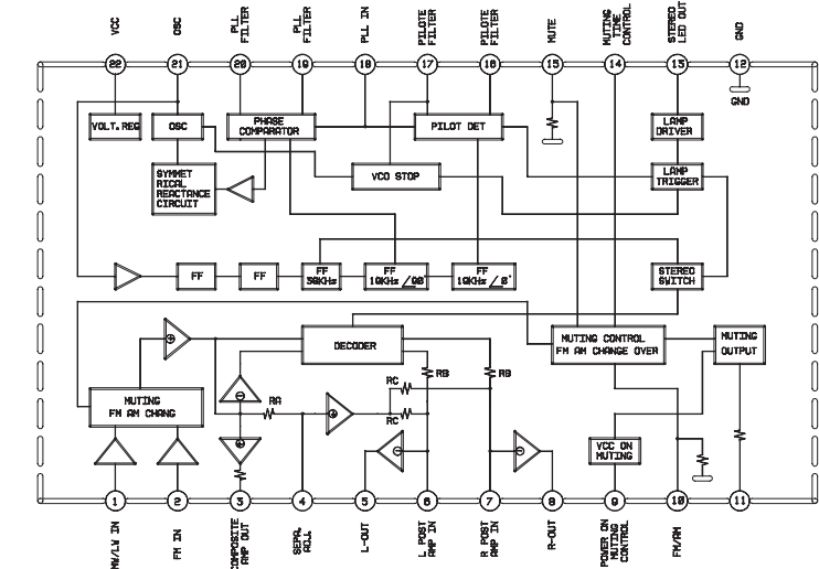
IC31 : LA3401
